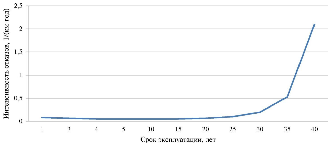
Рис. 8.1 - Интенсивность отказов в зависимости от срока эксплуатации участка тепловой сети
