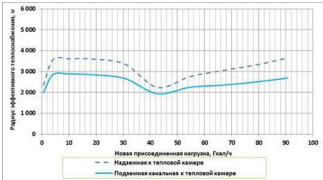
Рисунок 5.3 - Влияния способа прокладки на эффективный радиус
